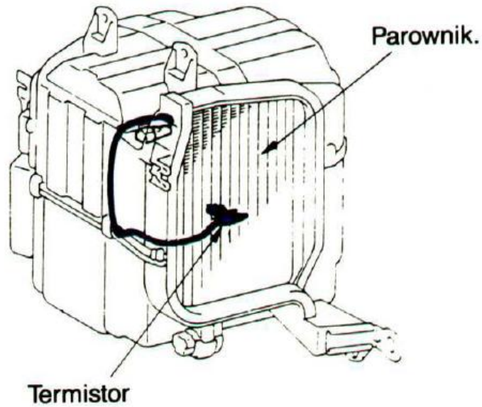
Rys. 7. Parownik i umieszczony na jego rdzeniu termistor
