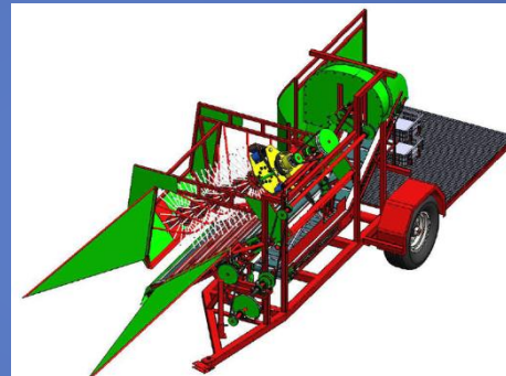
Źródło: Sumacz P., Projekt koncepcyjny kombajnu do zbioru porzeczki, praca inżynierska 2018
